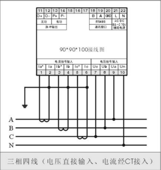
三相四线（电压直接输入、电流经CT接入）
