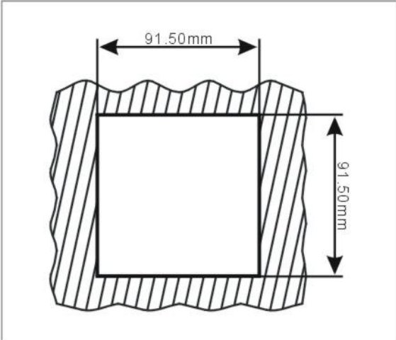
开孔尺寸:91.5*91.5（mm）
