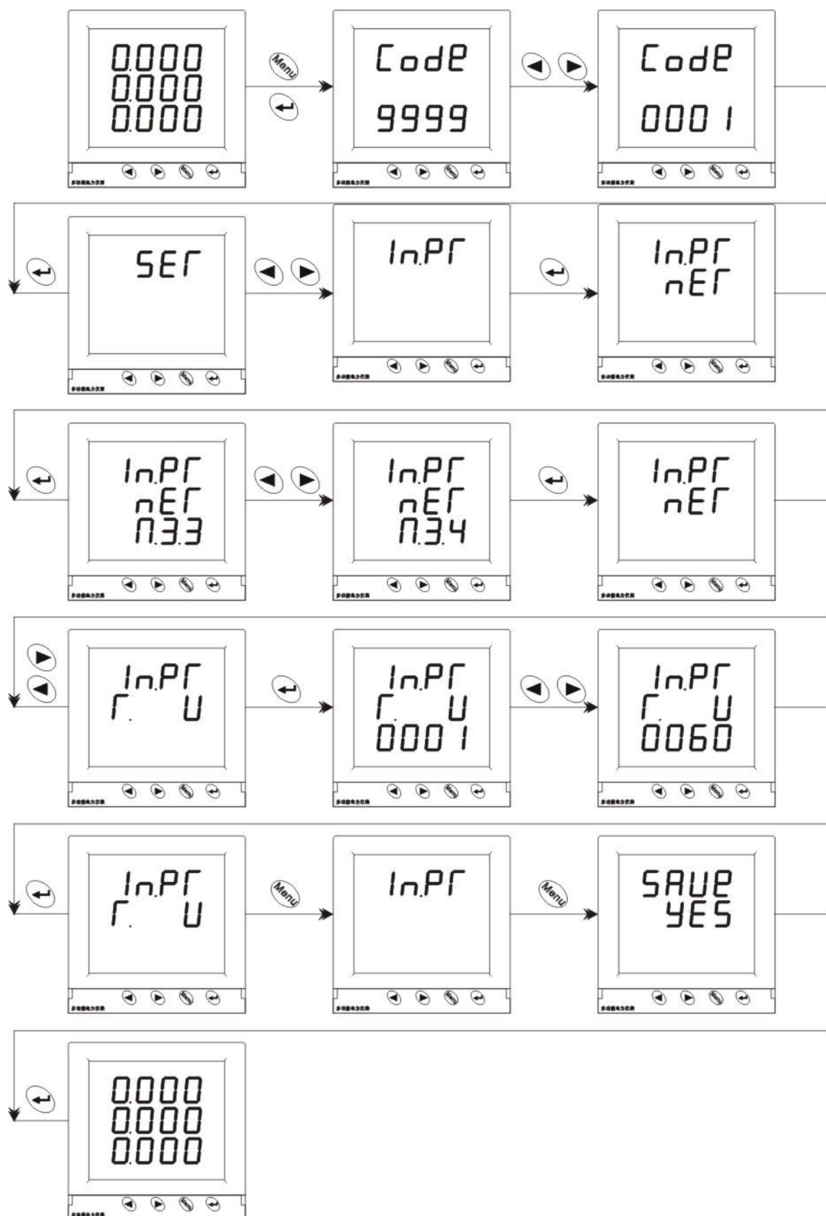
例 1：电压变比调试（例：10KV/100V）
