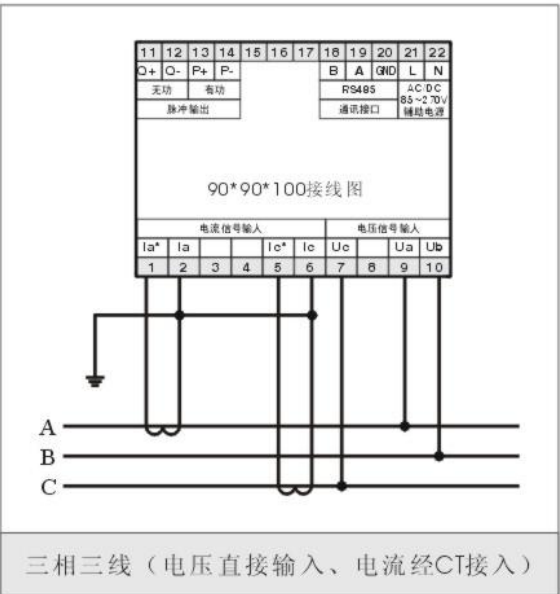
三相三线（电压直接输入、电流经CT接入）
