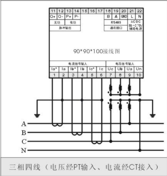
三相四线（电压经PT输入、电流经CT接入）
