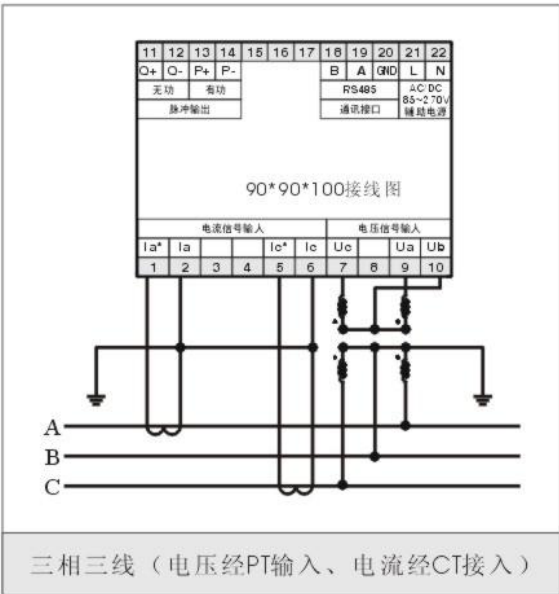
三相三线（电压经PT输入、电流经CT接入）
