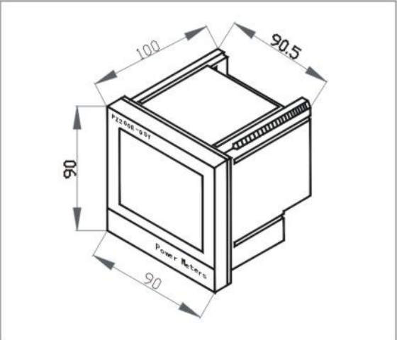
外形尺寸:90*90*100（mm）
